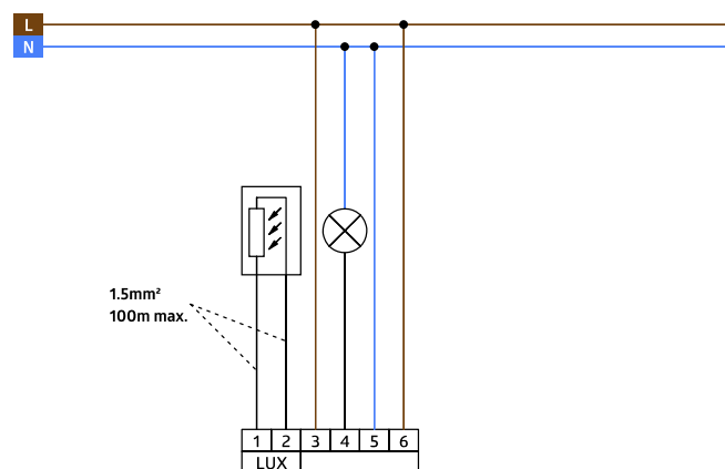
Kapcsolási rajzok
